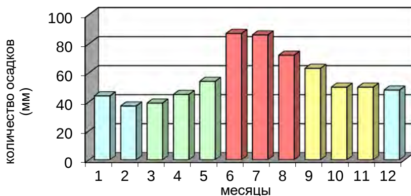
Рисунок 3.1 – Годовой ход осадков на территории исследований
