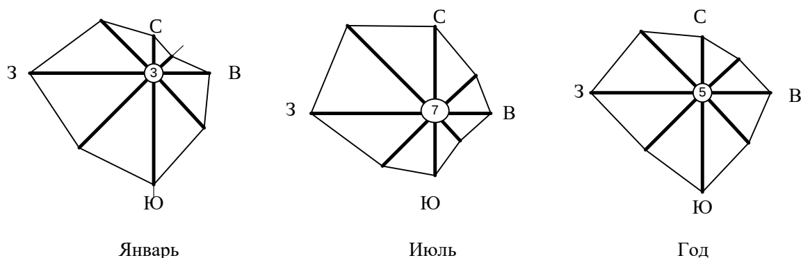
Рисунок 3.2 – Роза ветров района планируемой деятельности
