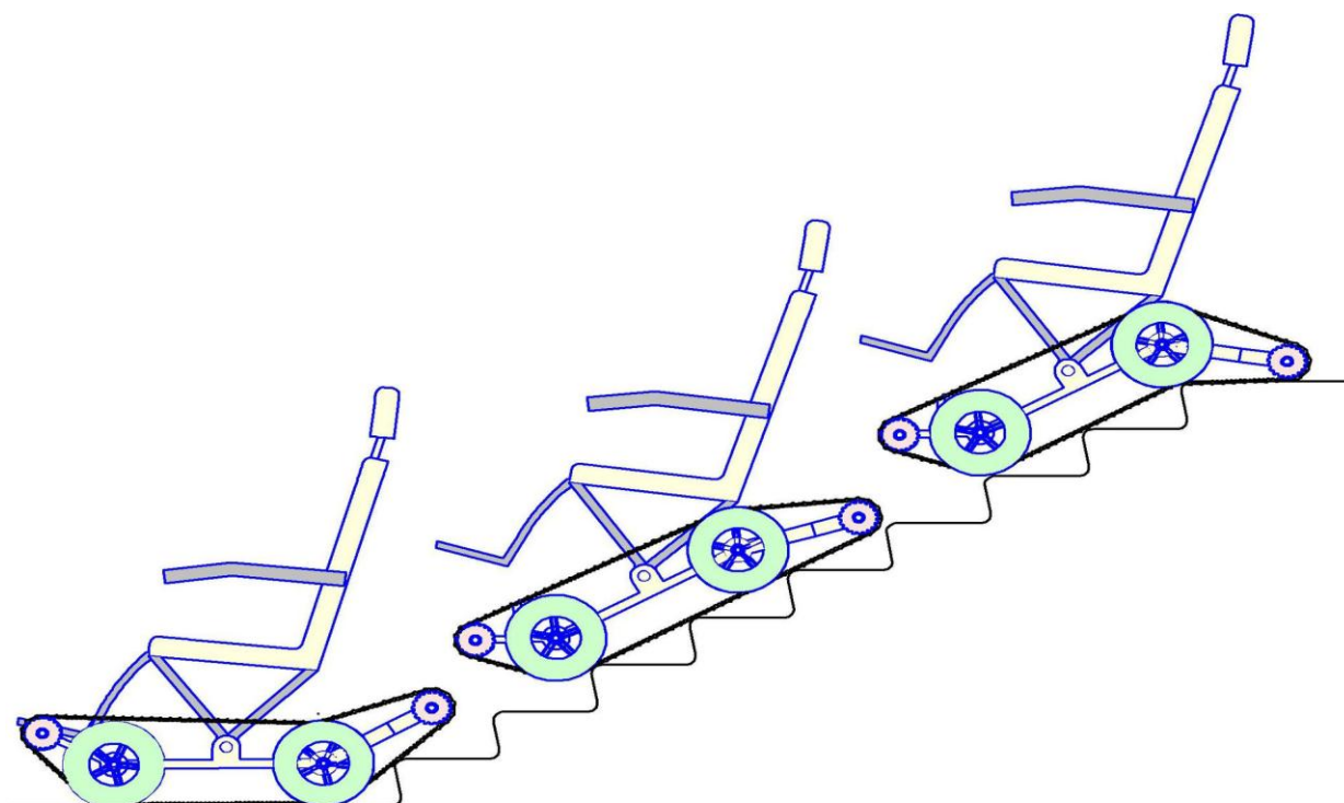
Коляска для передвижения по лестнице (рис 1)
